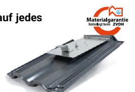
Im Bild: Rückseitig lastabtragende Stahlplatte mit Z-Profil zur Windsog-sicherung
